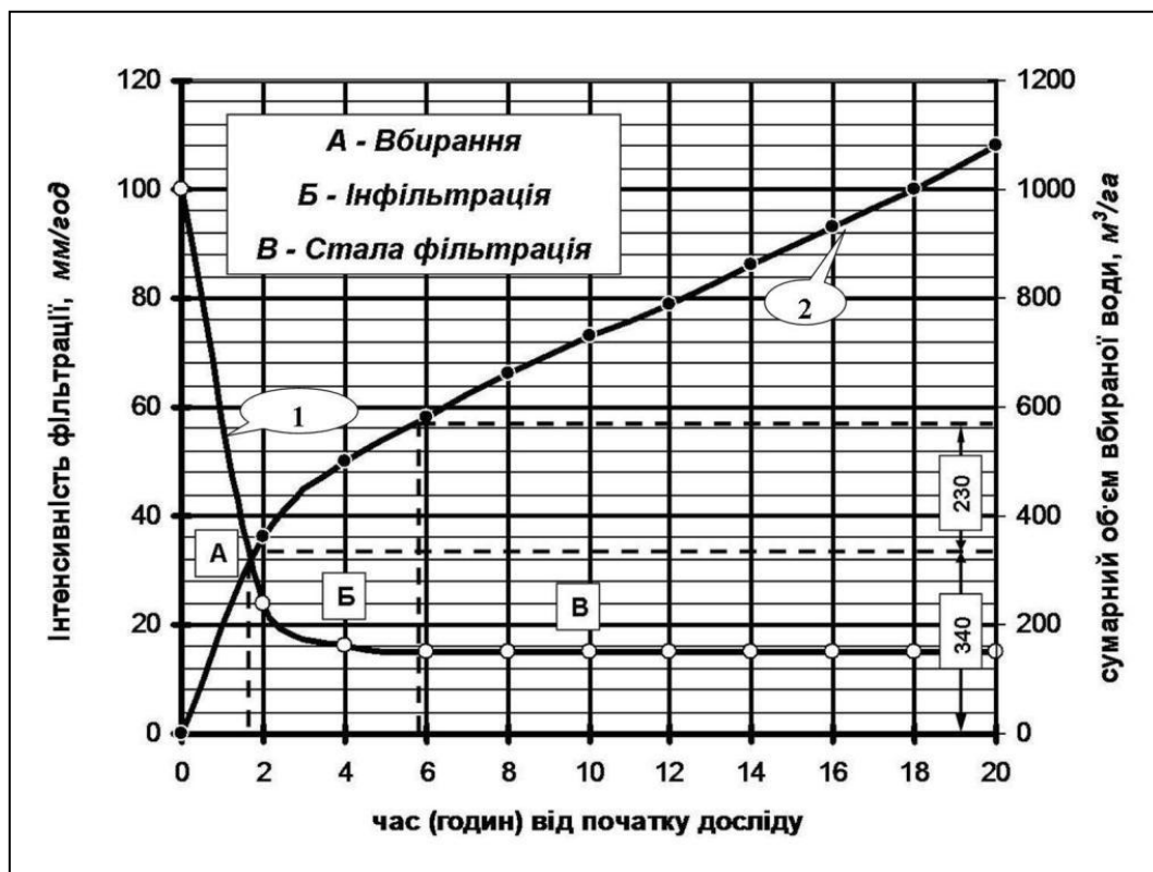
Рис. 4. Графік інтенсивності вбирання (А), інфільтрації (Б) і сталої фільтрації (В) води в ґрунт.
