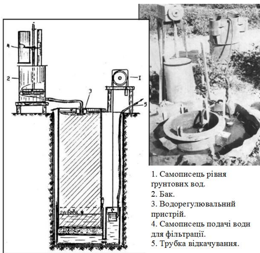
Рис. 3. Полева установка для вивчення швидкості фронту промочування, сталої фільтрації і водовіддачі із зони аерації ґрунтів (модернізований лізиметр ГР-80).
